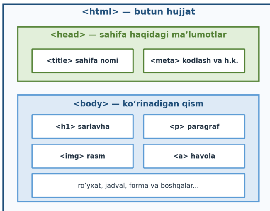
4-rasm. HTML hujjatning umumiy tuzilmasi
