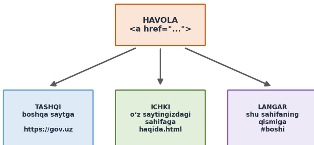
7-rasm. Havolalarning asosiy turlari
